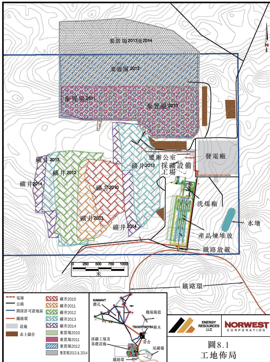
圖8.1 工地佈局
